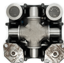
SPICER CRUCETA DE DADOS PAREJOS 18 44,000 LBS 5-281X
